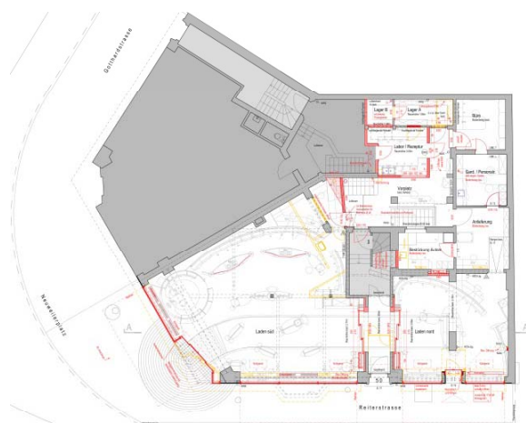
Grundriss Erdgeschoss bestehend / abbruch / neu
