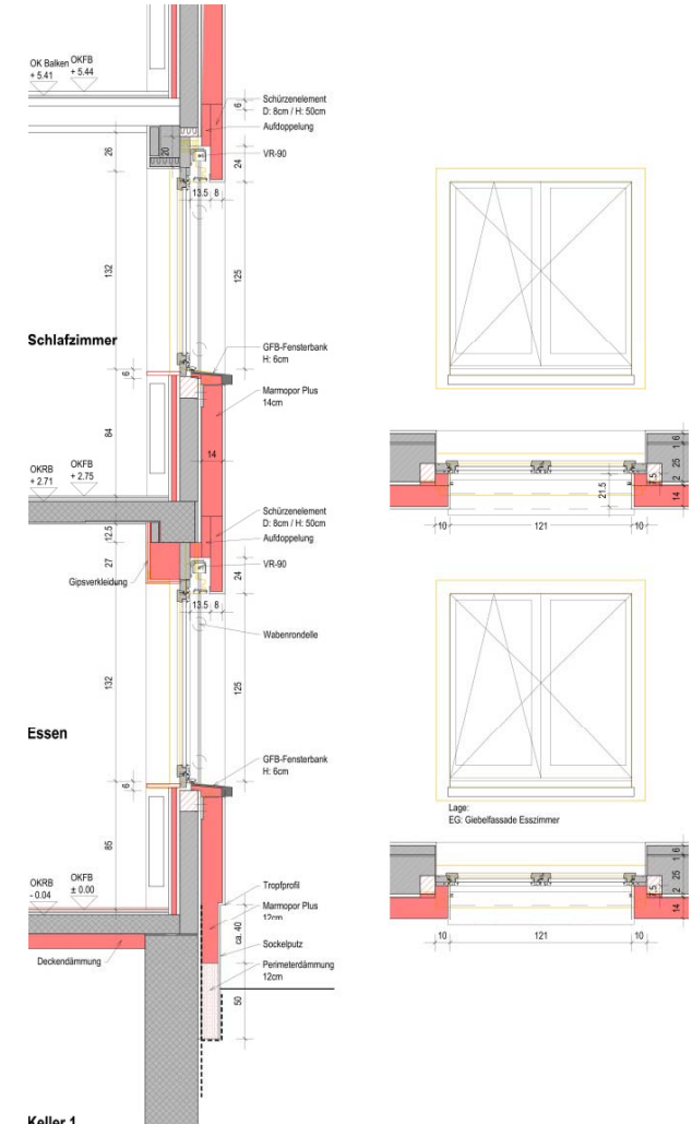
Fassadenschnitt, Fensteransichten und Fenster im Grundriss
