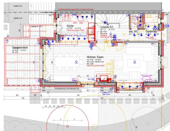
Erdgeschoss bestehend / abbruch / neu
