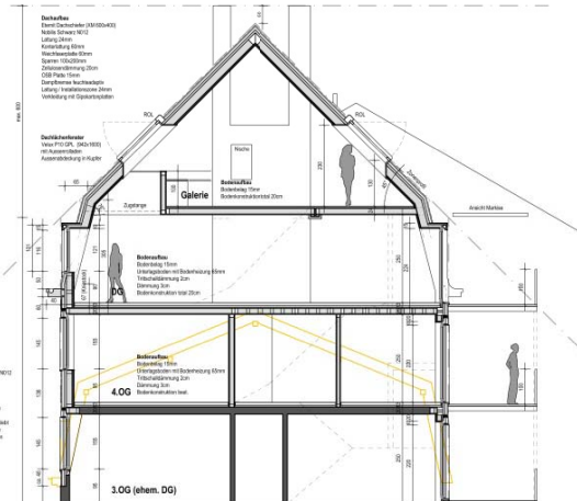
Schnitt durch das neue Dachgeschoss
