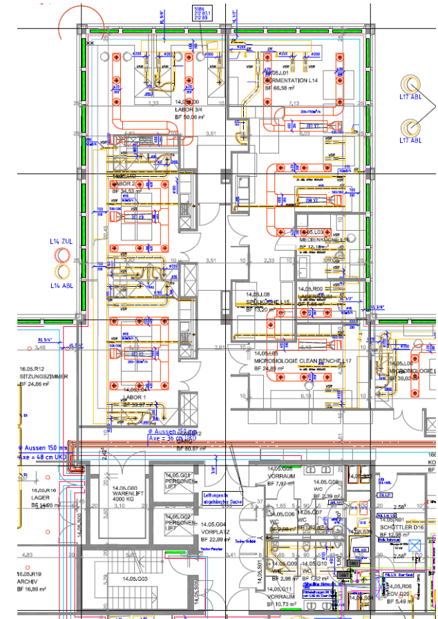
Ausschnitt Grundriss 5. OG, Koordinationsplan Haustechnik
