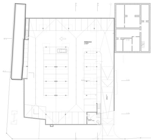
Untergeschoss Parkhaus
