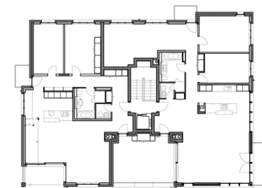
2. Obergeschoss
