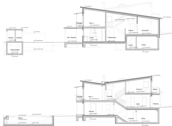
Schnitte. Split-level
